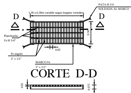
REJILLA TIPO
