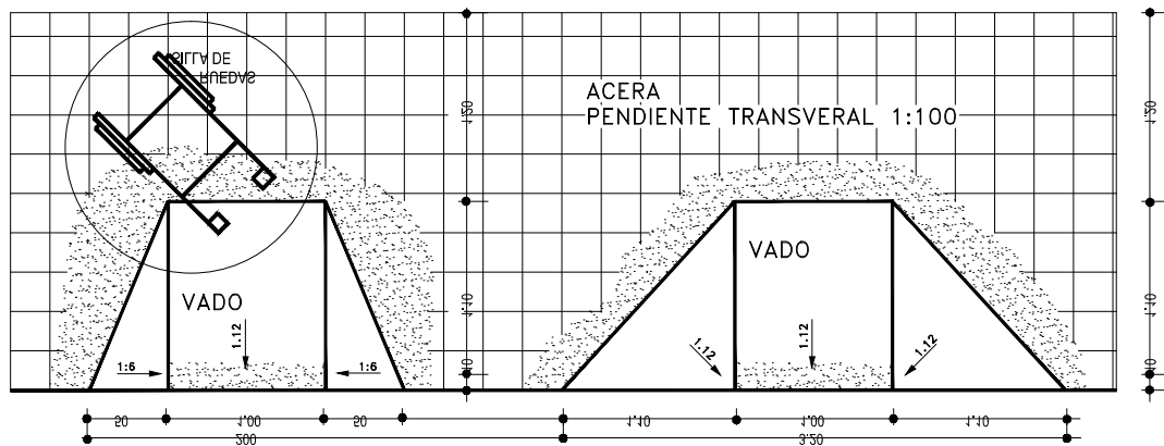
PLANTA
