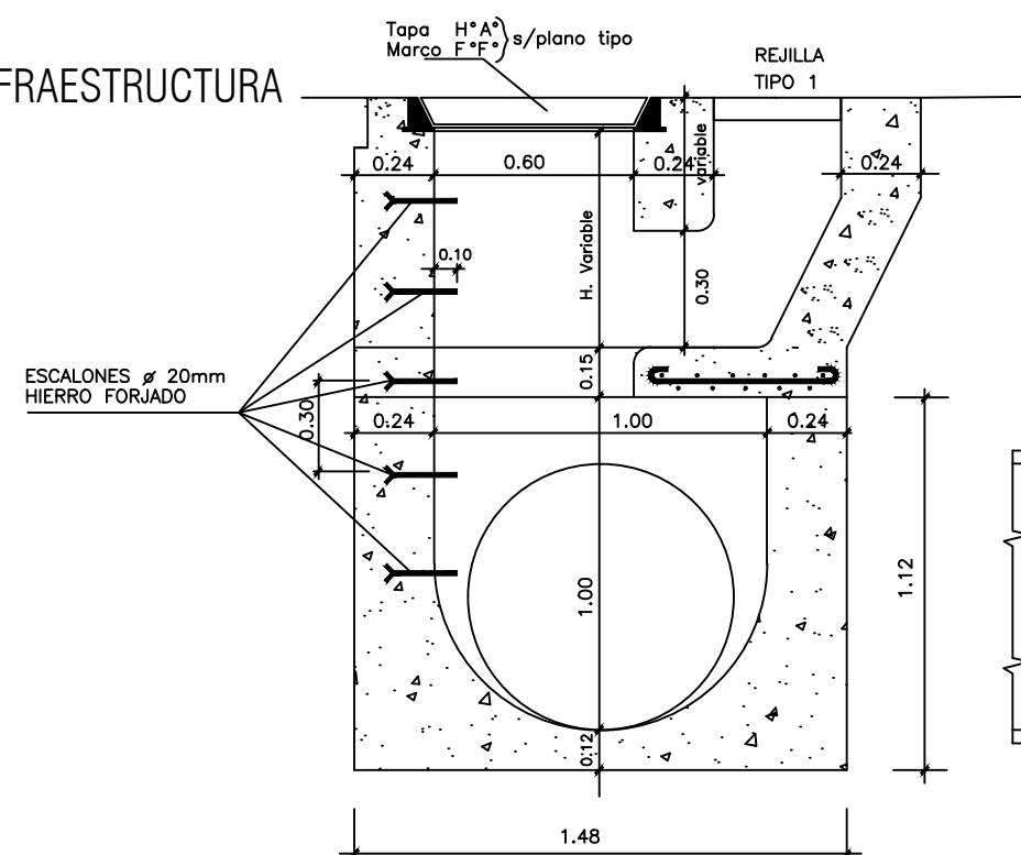
CORTE A-A
