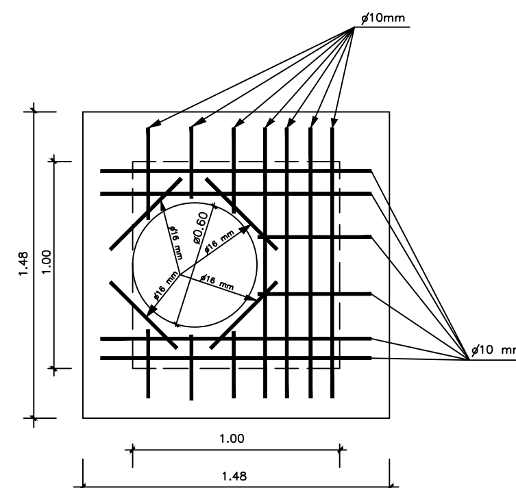
DISTRIBUCION DE LA ARMADURA DE LA LOSA
