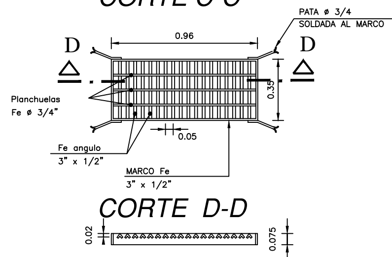
REJILLA TIPO 1 CORTE C-C
