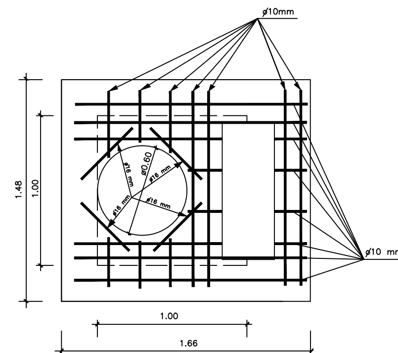
DISTRIBUCION DE LA ARMADURA DE LA LOSA
