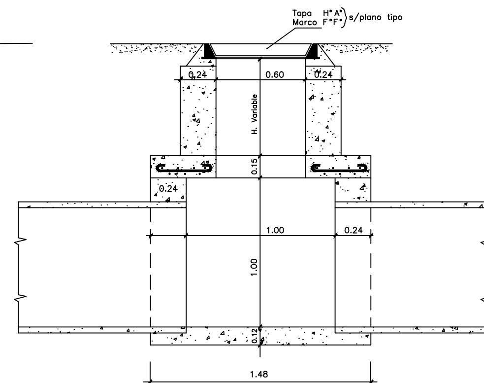
CORTE B-B
