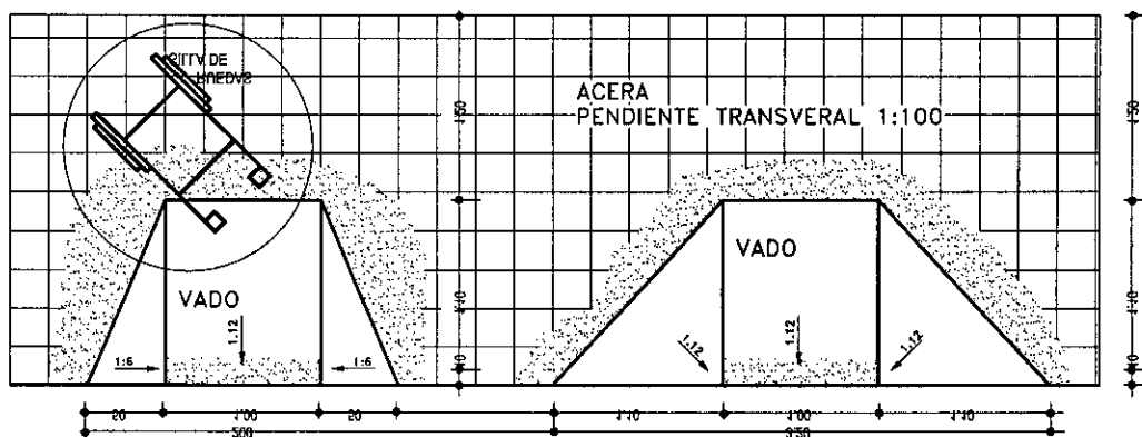
PLANTA
