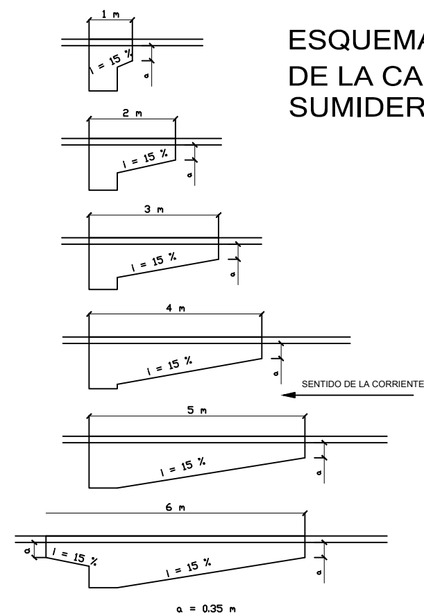
MODIFICACION DE PAVIMENTO PARA FORMACION DE HOYA
