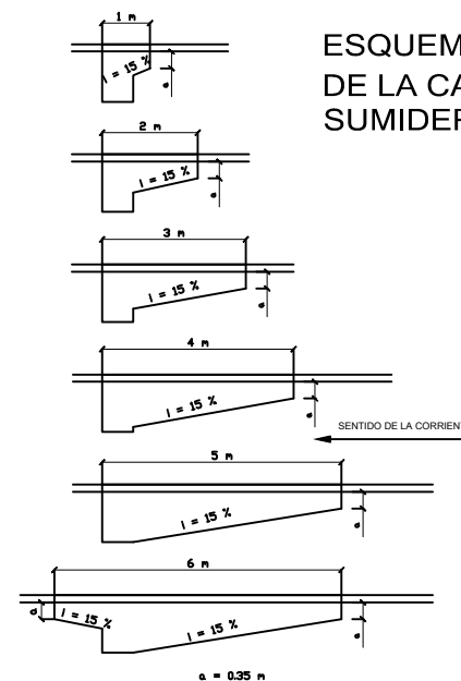
MODIFICACION DE PAVIMENTO PARA FORMACION DE HOYA
