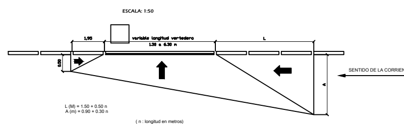
MODIFICACION DE PAVIMENTO PARA FORMACION DE HOYA
